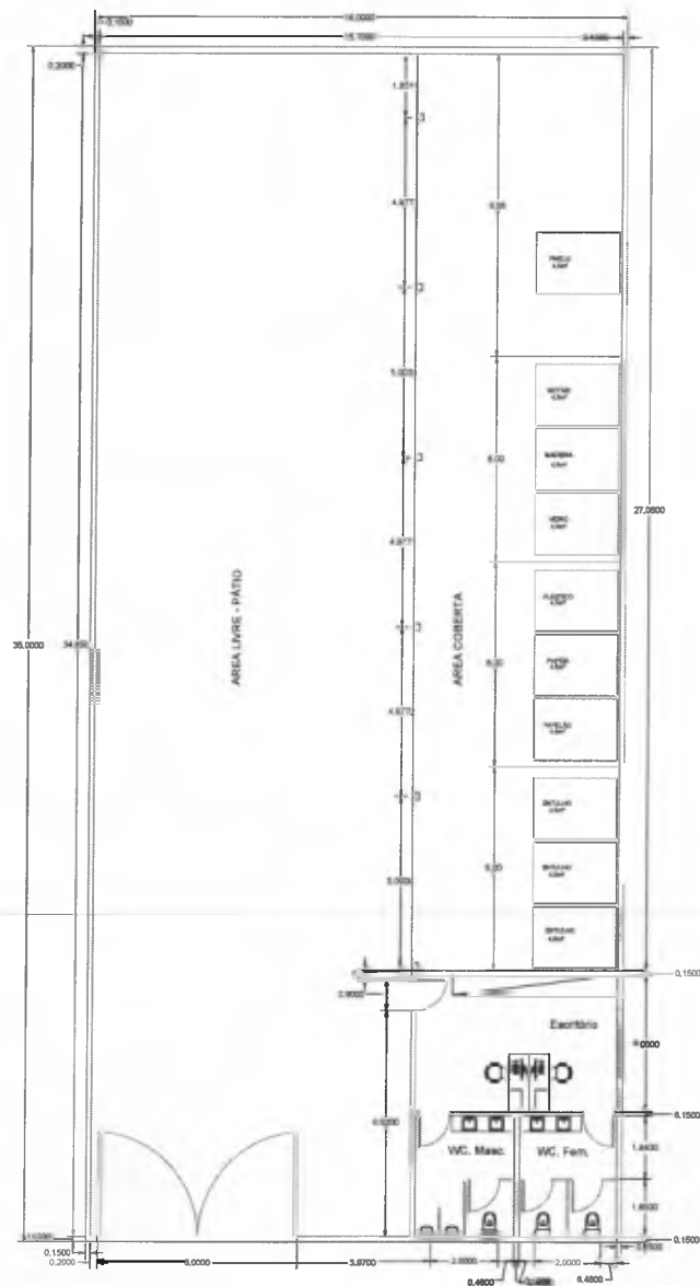
PLANTA BAIXA - ECOPONTO ESC. 1/100
